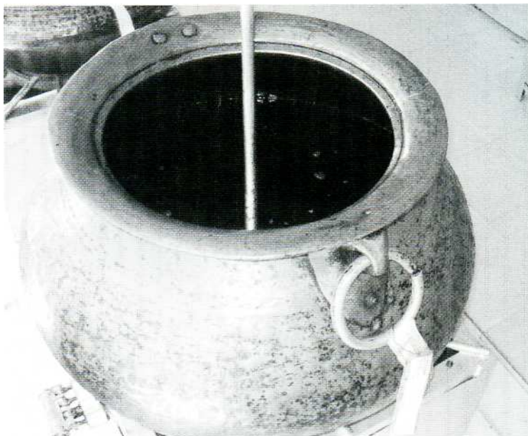
Abb. 83: Kupferkessel zur Ölherstellung
